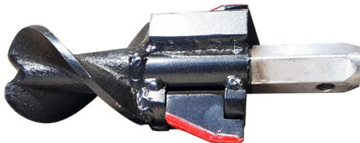
Głowica nożowa dla średnic \varnothing 90 , \varnothing 110 , \varnothing 130 , \varnothing 170 , \varnothing 230
