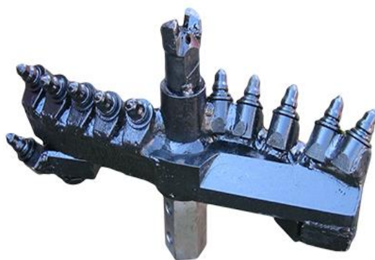
Głowica widiowa dwuramienna dla średnic od \varnothing 215 do \varnothing 560
